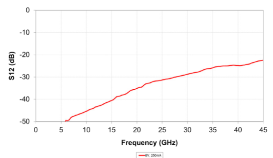
S12
