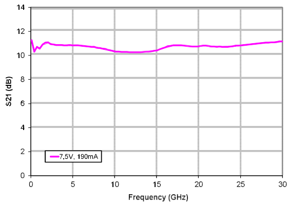
S21
