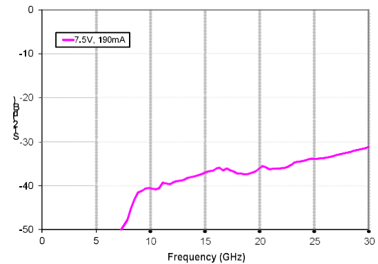
S12
