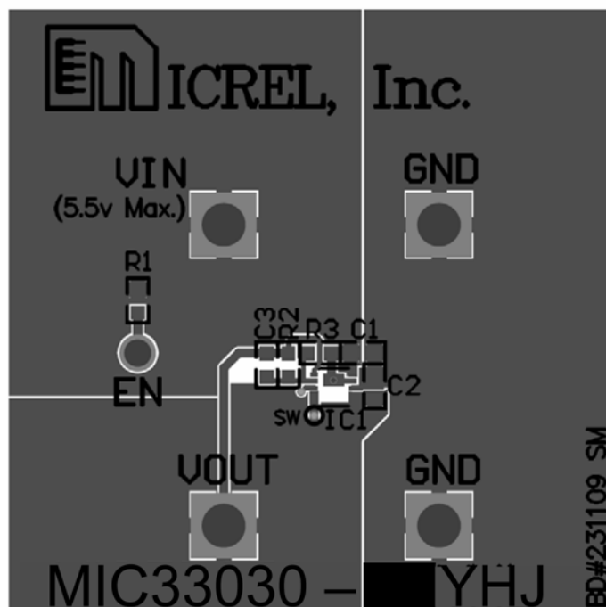
MIC33030 EVB Top Layer
