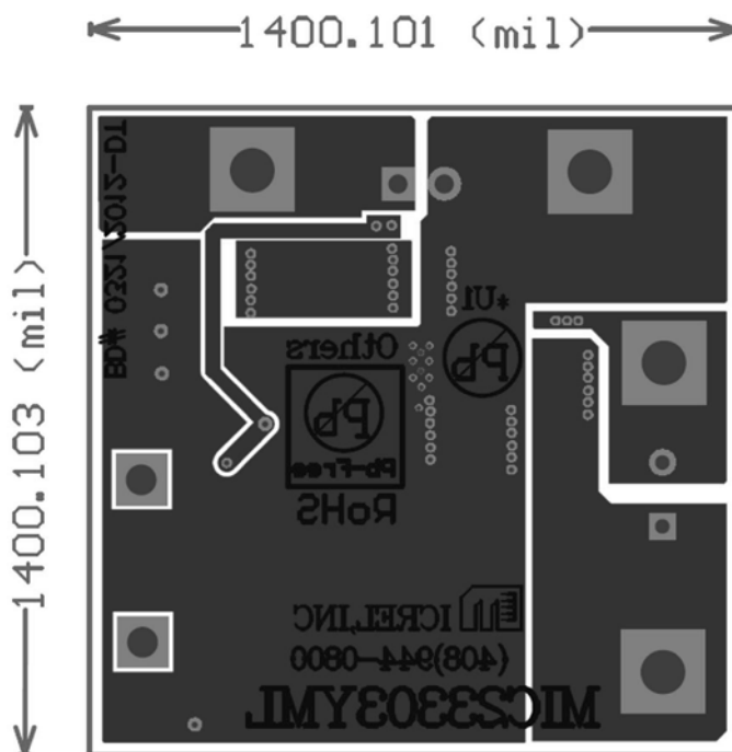
Bottom Layer
