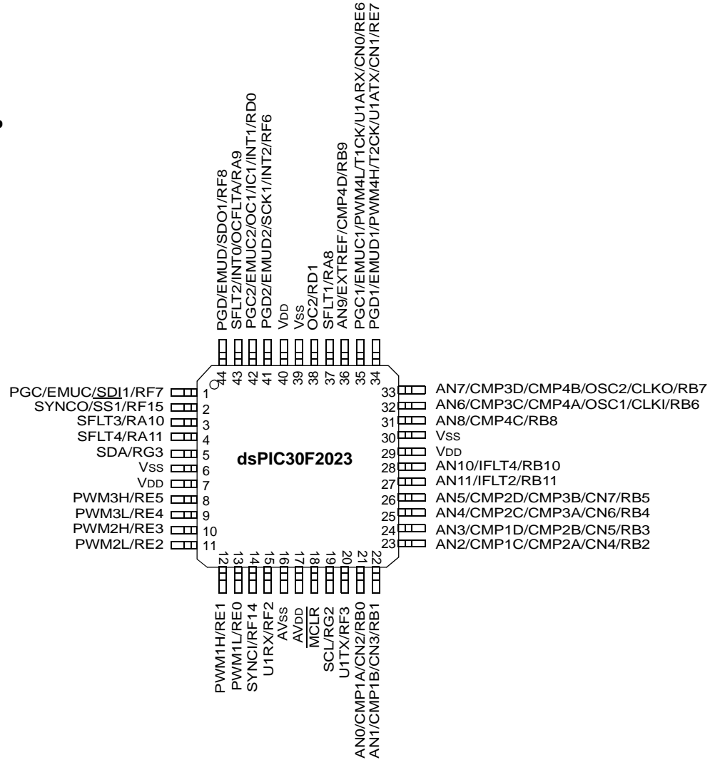
44-Pin TQFP
