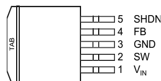
5-Pin TO-263 (U)
