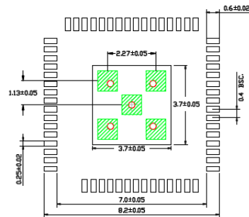
RECOMMENDED LAND PATTERN NOTE : 8,9
