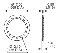
LOCKWASHER
