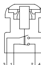
Function 8 (NC/NO))
