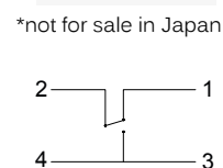
NC/NO function
