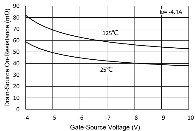
Fig.3 R_{DS(on)} - V_{GS}
