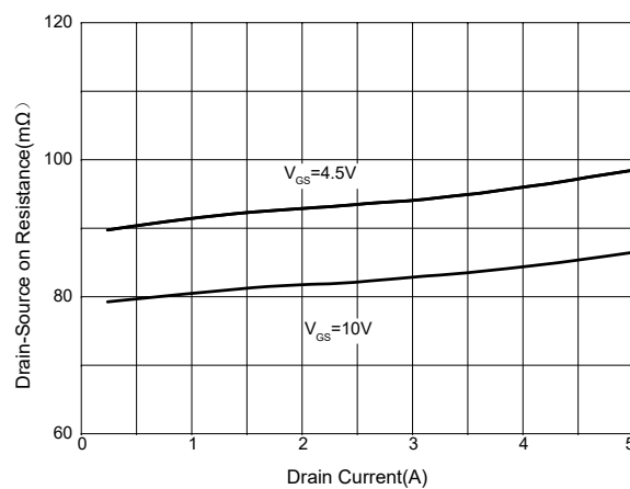
Fig. 4 - R_{DS(ON)} - I_D
