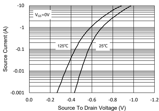
Fig.9 - I_S - V_{SD}
