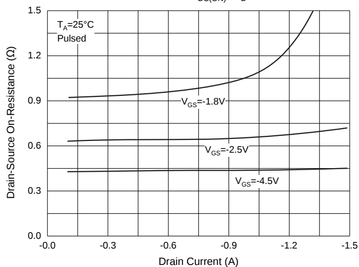
Fig. 3 - R_{DS(ON)} - I_D
