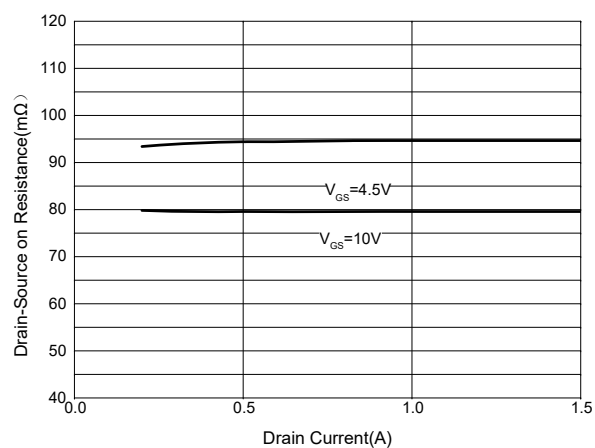
Fig. 4 - R_{DS(ON)} - I_D
