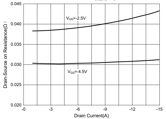
Fig. 4 - R_{DS(ON)} - I_D
