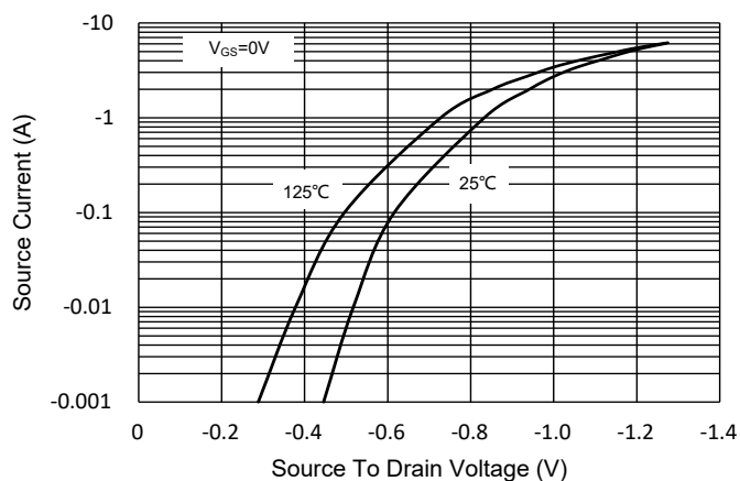
Fig.9 - I_S - V_{SD}
