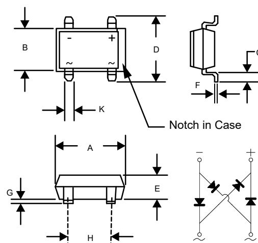
DIMENSIONS
