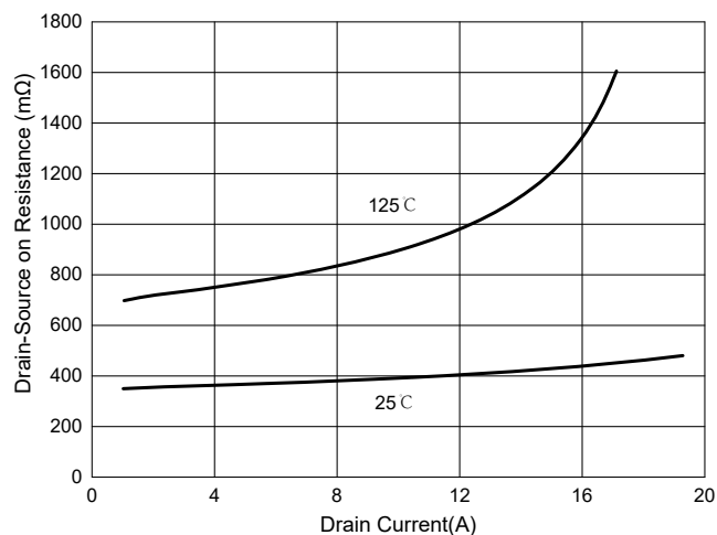
Fig. 7 - R_{DS(ON)} - I_D
