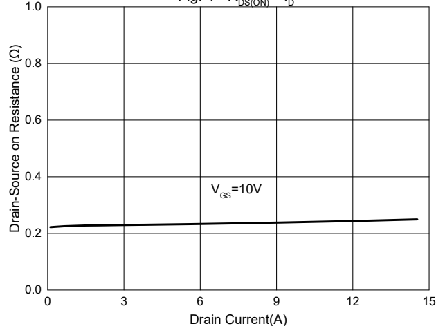
Fig. 4 - R_{DS(ON)} - I_D
