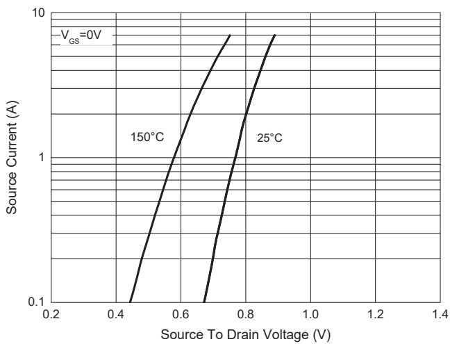
Fig. 9 - I_S - V_{SD}
