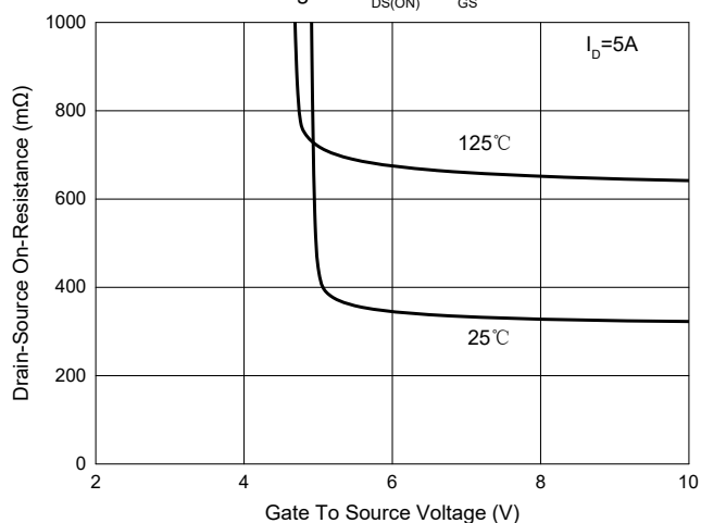
Fig. 3 - R_{DS(ON)} - V_{GS}
