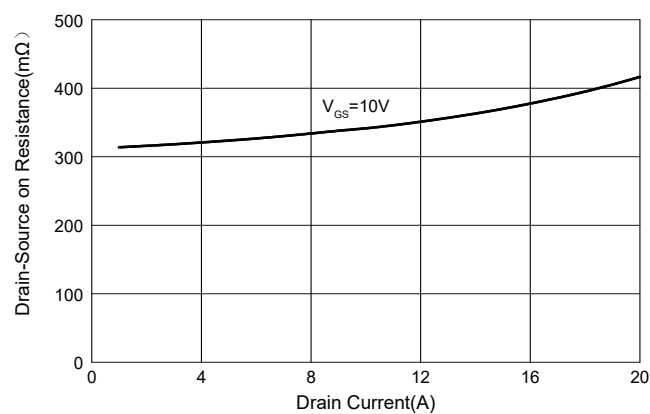
Fig.4 - R_{DS(ON)} - I_D
