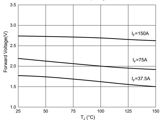
Fig. 8 - V_F - T_J
