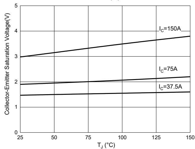
Fig. 4 - V_{CE(sat)} - T_J
