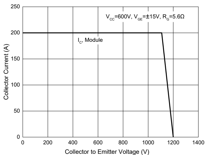
Fig. 5 - RBSOA
