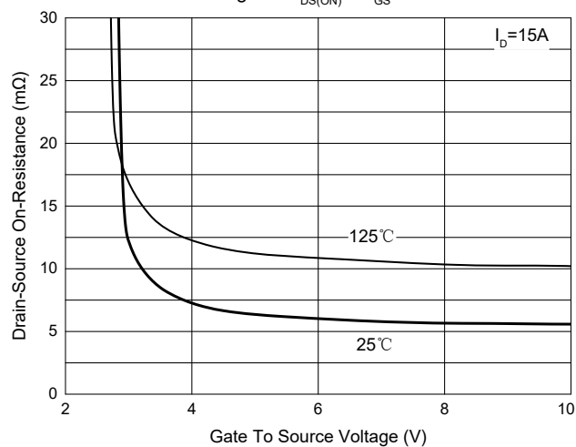
Fig. 3 - R_{DS(ON)} - V_{GS}
