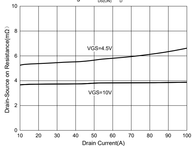
Fig. 4 - R_{DS(ON)} - I_D
