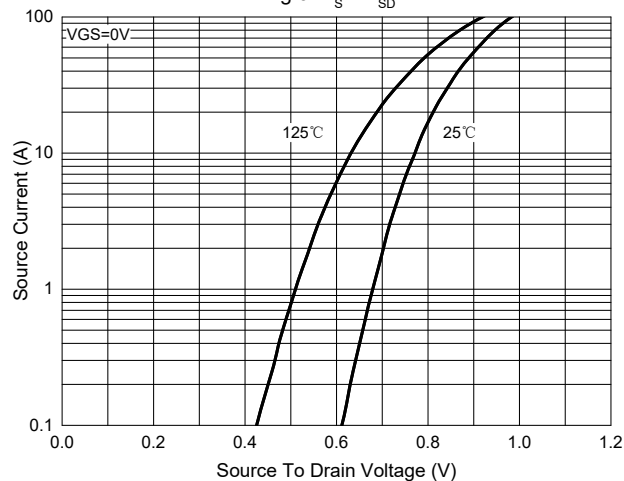
Fig.9 - I_S - V_{SD}
