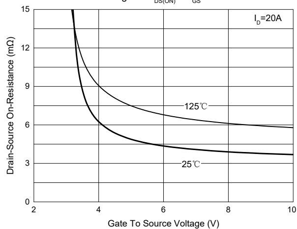
Fig. 3 - R_{DS(ON)} - V_{GS}
