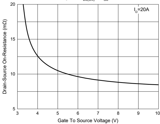
Fig. 3 - R_{DS(ON)} - V_{GS}
