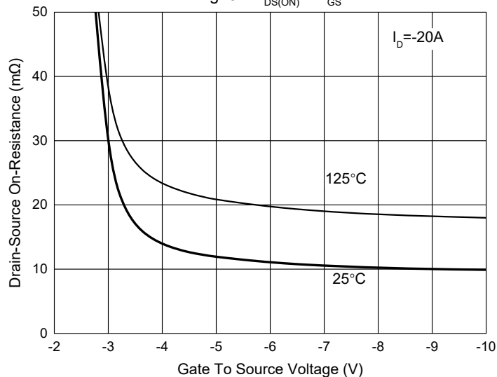
Fig. 3 - R_{DS(ON)} — V_{GS}
