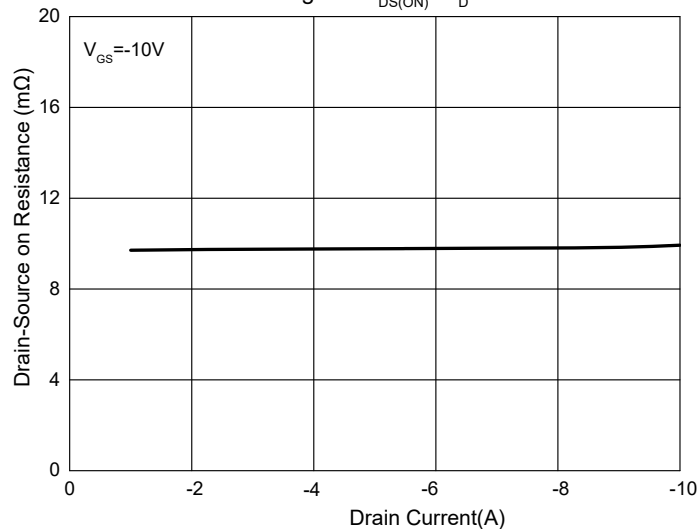
Fig. 4 - R_{DS(ON)} — I_D
