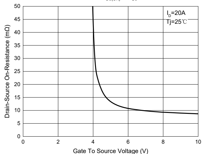
Fig. 7 - R_{DS(ON)} - V_{GS}
