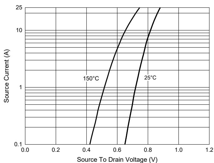
Fig. 9 - I_S - V_{SD}
