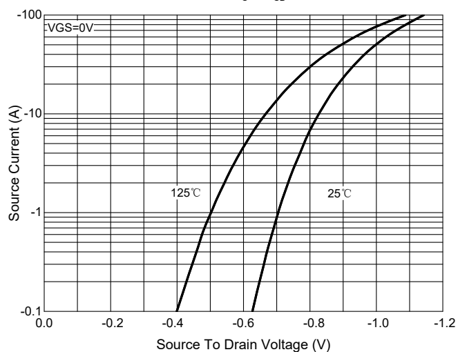
Fig.9 - I_S - V_{SD}
