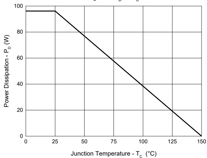
Fig. 10 - P_D - T_C
