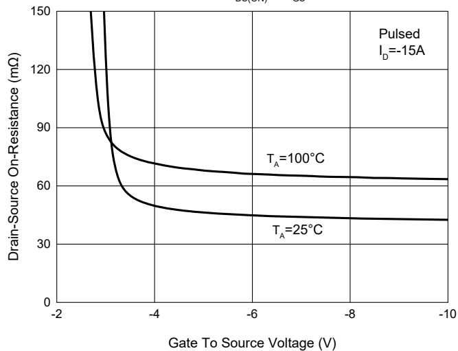
Fig. 5 - R_{DS(ON)} - V_{GS}
