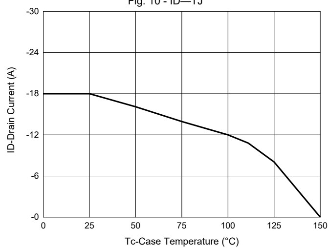
Fig. 10 - I_D - T_J
