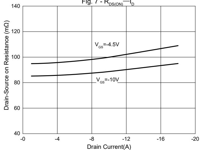
Fig. 7 - R_{DS(ON)} - I_D
