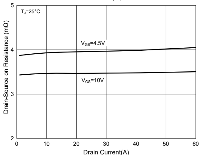
Fig. 5 - R_{DS(ON)} - I_D
