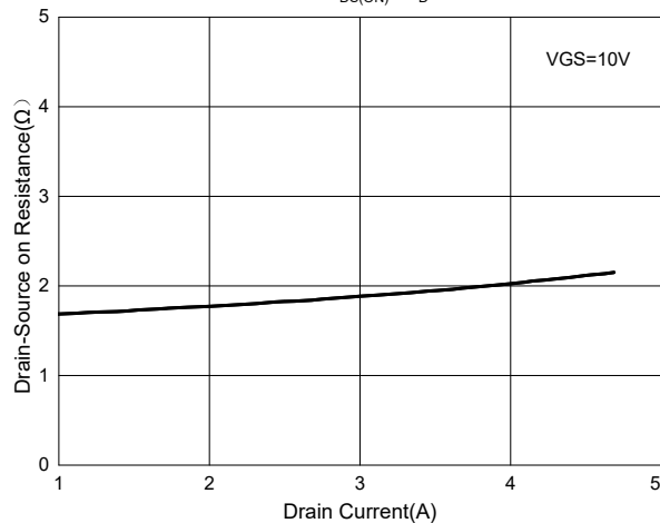
Fig. 4 - R_{DS(ON)} - I_D
