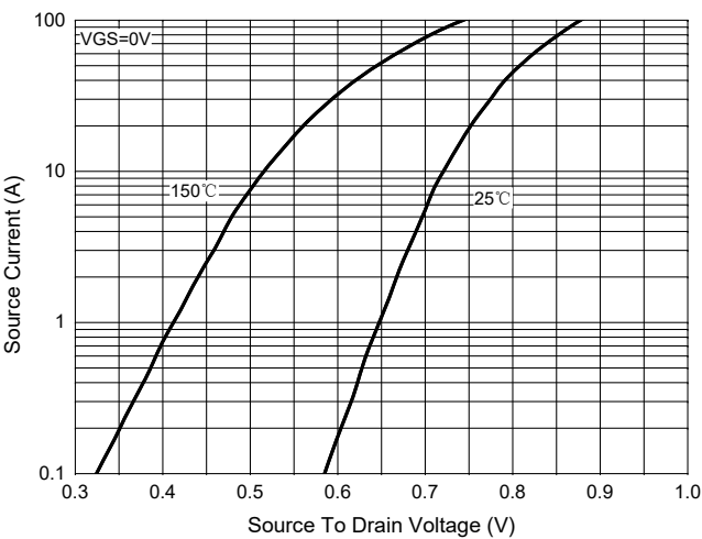
Fig. 9 - I_S-V_{SD}
