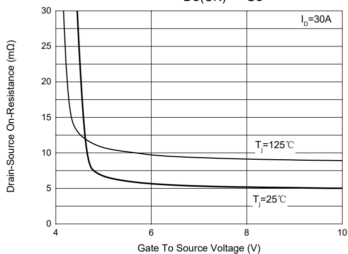
Fig. 3 - R_{DS(ON)} - V_{GS}
