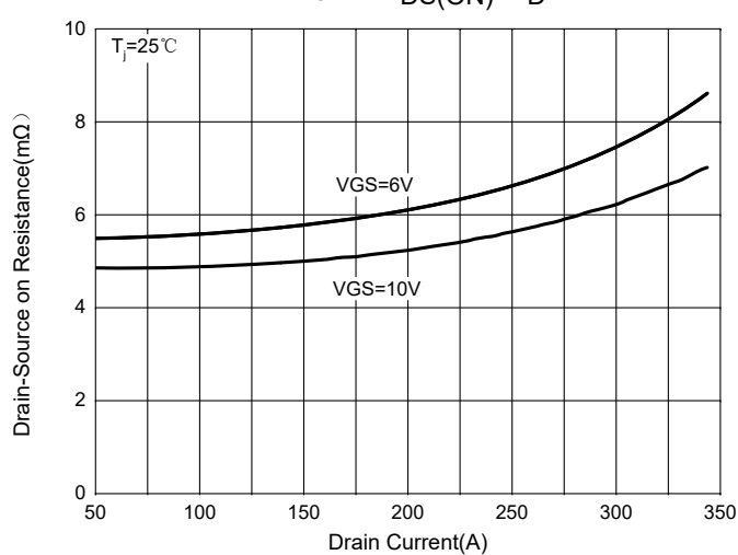
Fig. 4 - R_{DS(ON)} - I_D
