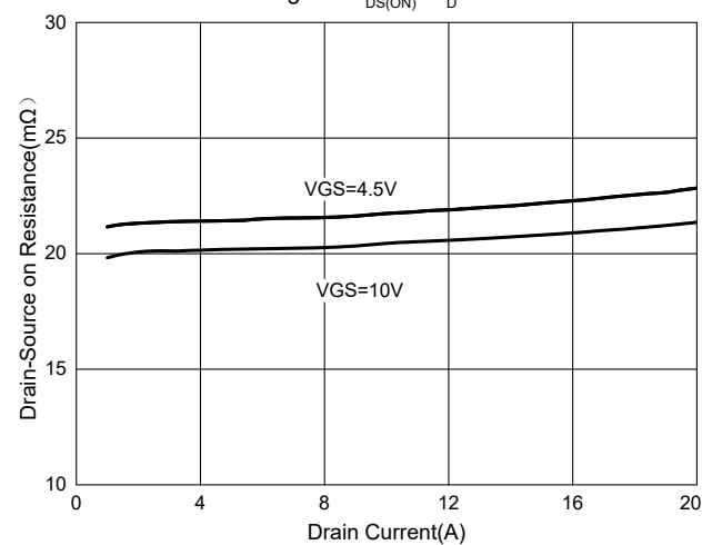
Fig. 4 - R_{DS(ON)} - I_D
