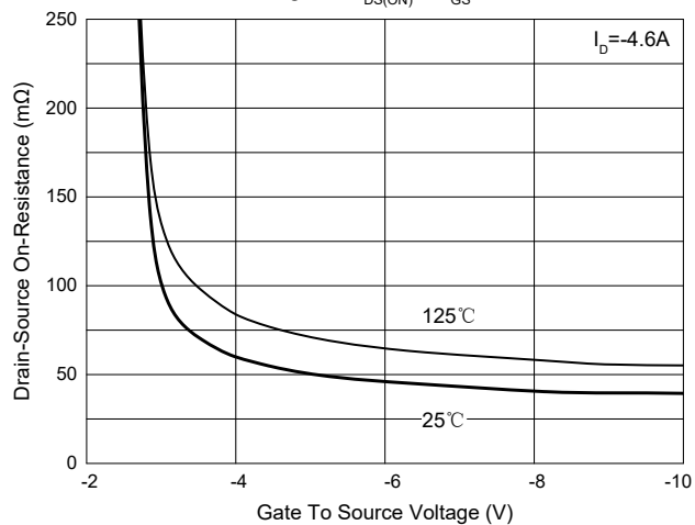
Fig. 3 - R_{DS(ON)} - V_{GS}
