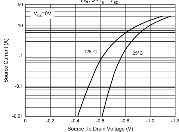
Fig. 9 - I_S - V_{SD}
