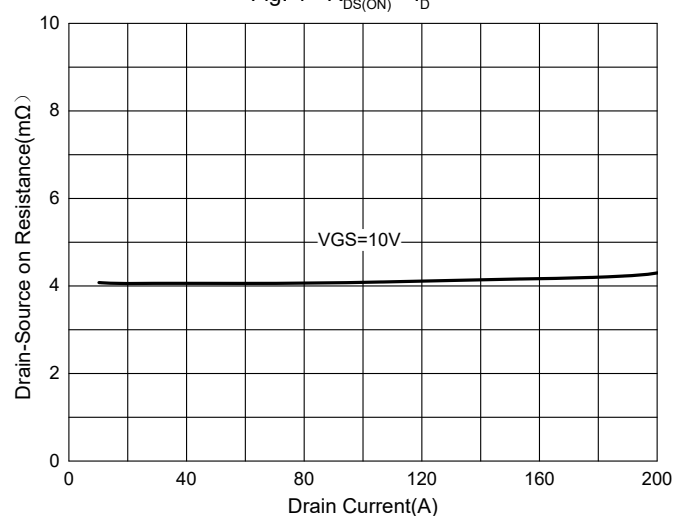
Fig. 4 - R_{DS(ON)} - I_D
