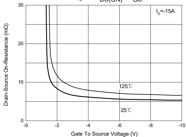
Fig. 3 - R_{DS(ON)}-V_{GS}
