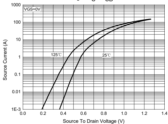
Fig.9 - I_S - V_{SD}
