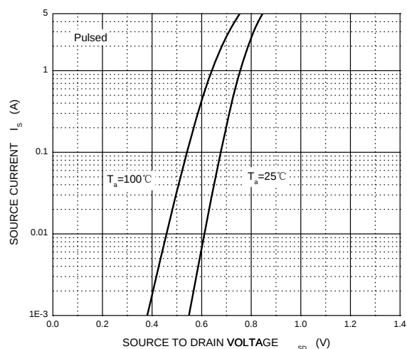
Fig. 5 - I_S-V_{SD}
