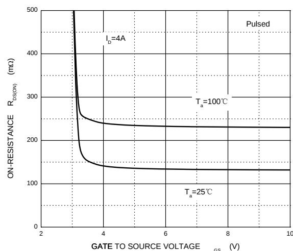
Fig. 4 - R_{DS(ON)}-V_{GS}
