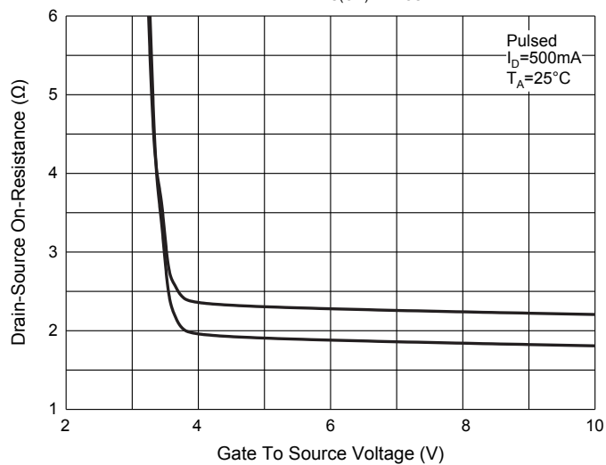
Fig. 4 - R_{DS(ON)} - V_{GS}
