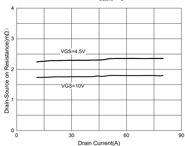
Fig. 4 - R_{DS(ON)} - I_D
