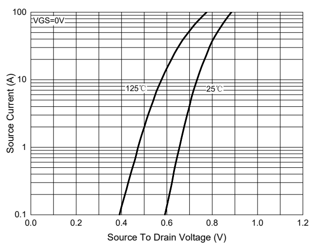
Fig.9 - I_S - V_{SD}
