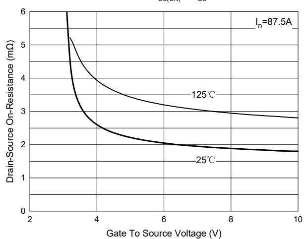
Fig. 3 - R_{DS(ON)} - V_{GS}
