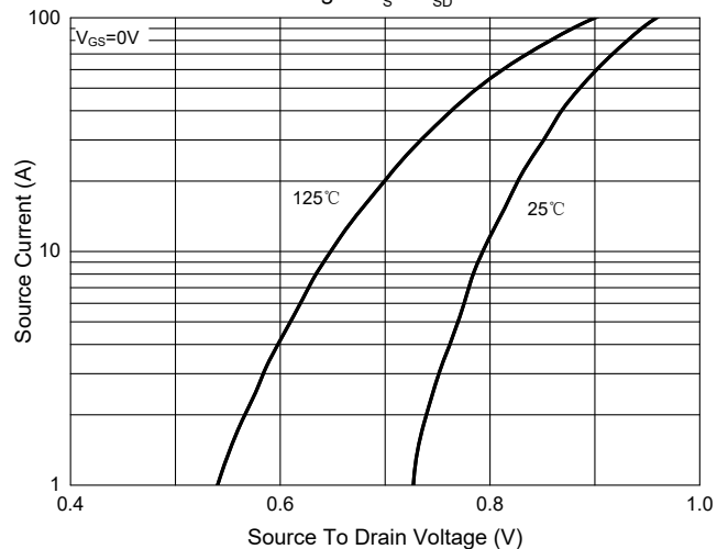
Fig.9 - I_S - V_{SD}
