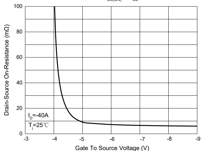
Fig. 8 - R_{DS(on)} - V_{GS}
