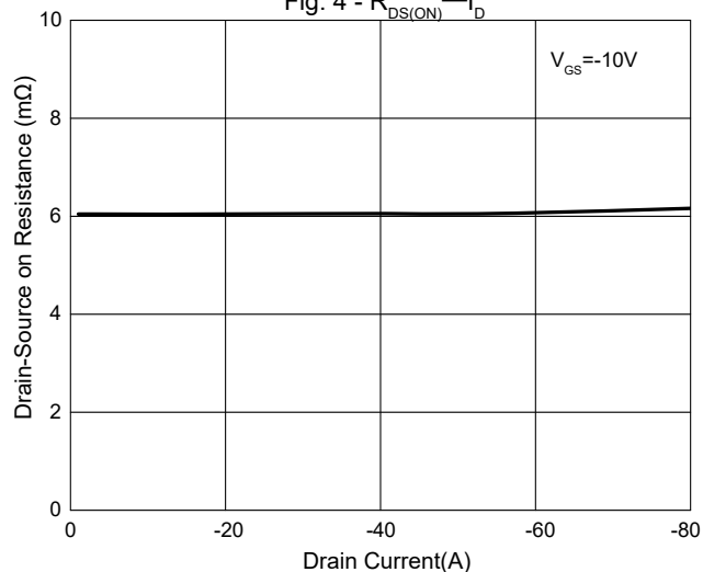
Fig. 4 - R_{DS(ON)} - I_D
