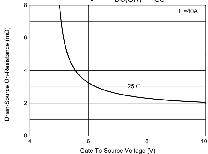
Fig. 3 - R_{DS(ON)}-V_{GS}
