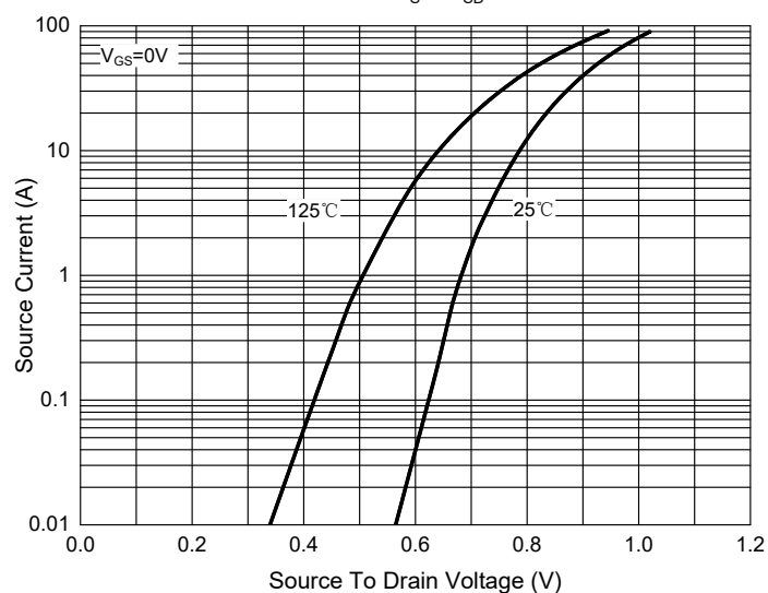
Fig.9 - I_S - V_{SD}
