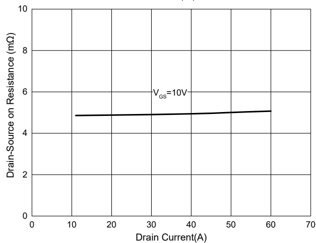
Fig. 4 - R_{DS(ON)} - I_D
